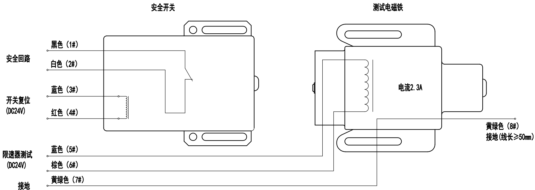
线号示意
