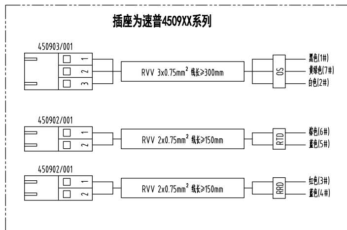
线号示意
