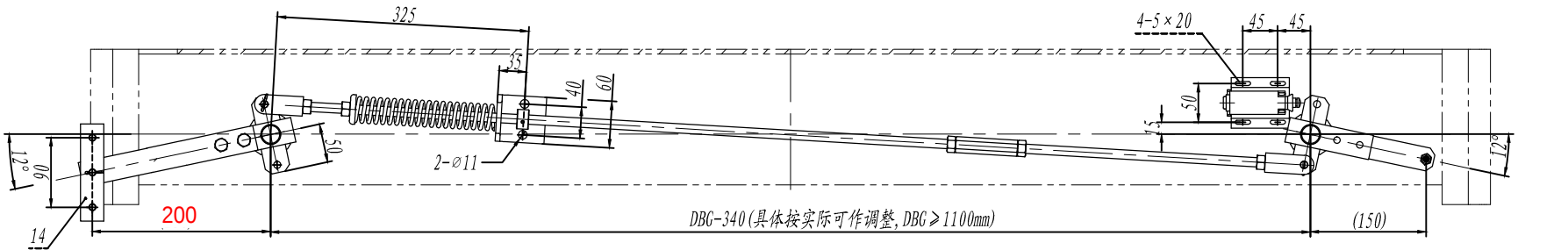
80013146 OX-188BT安全联动机构(提拉板孔距200)DBG=1540 C=220 L3=200 中英文 浙江富奥机电 P1-2
