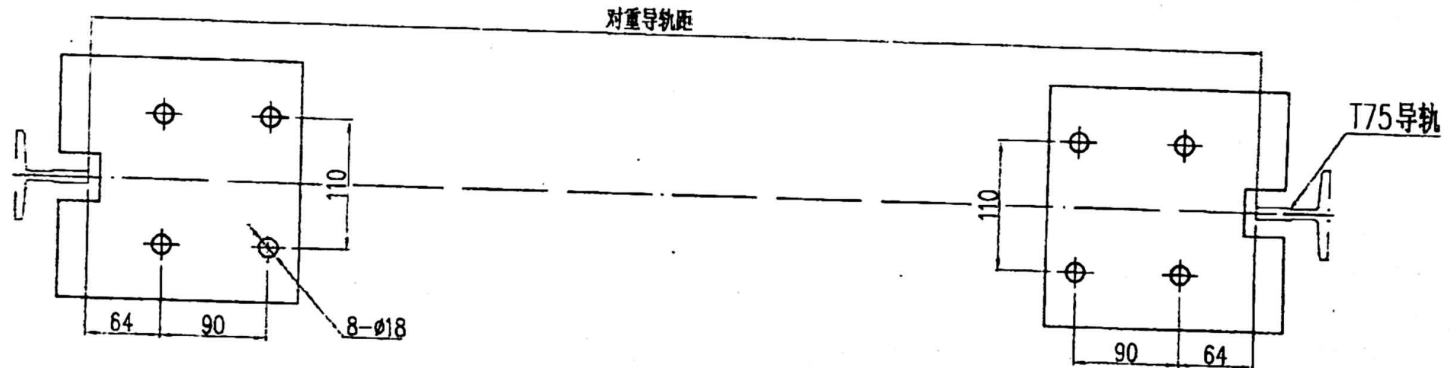
下部连接孔位示意图
