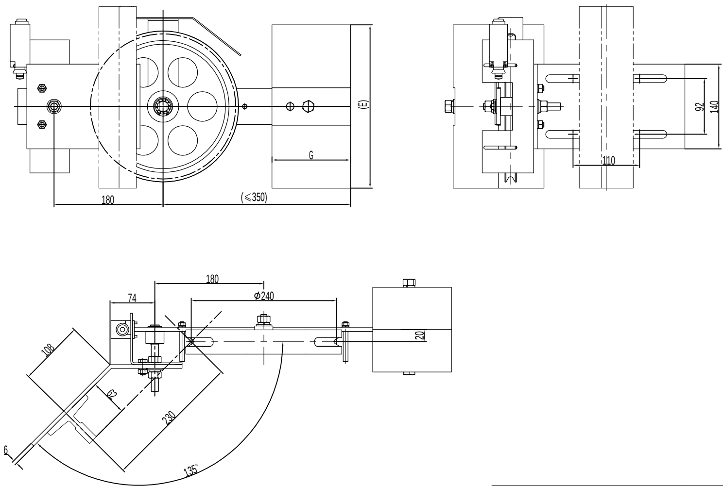
80011894 OX-200涨紧装置(240-135-230-0)240-8 重晶石12KG 本色RAL6005 中英文 歌拉瑞 P1-2
