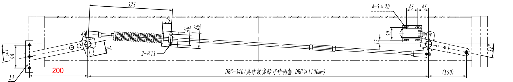
80011797 OX-188BT安全联动机构(提拉板孔距200)DBG=1690 C=220 L3=200 中英文 中都国脉 P1-2
