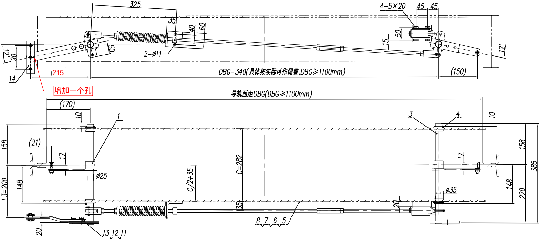
本装置适用单提拉结构形式。
