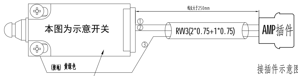
开关接线示意图
