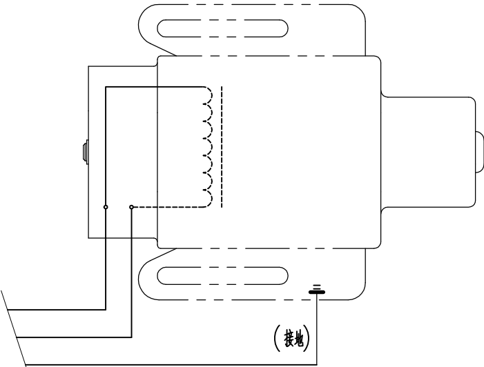
限速测试动作线图
