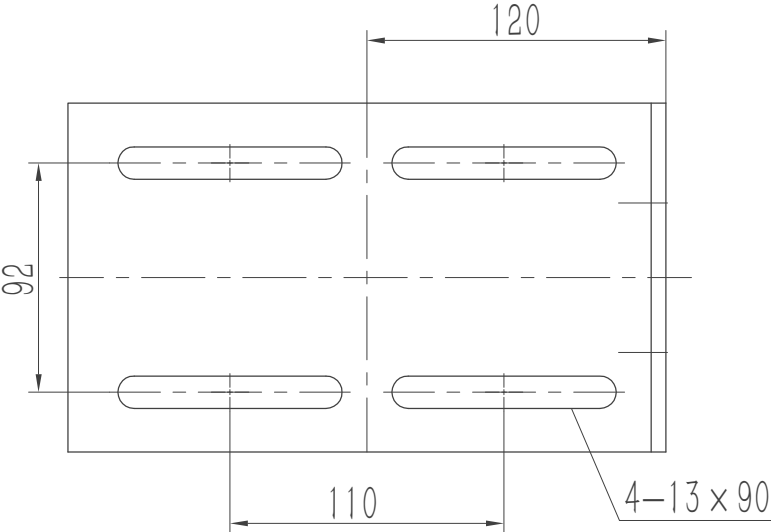
80010854 OX-200涨紧装置(240-90-155-28 导轨高度56) 240-8 铸铁12kg RAL6005本色 中英文 凯斯博 P2
