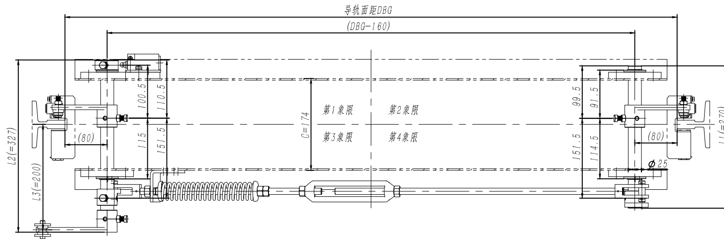
80010812 OX-210BTX 联动机构 (C=174,L3=200) DBG=1180(第二、三象限) 摇臂孔距105 中英文 海宁欧立 P1-2
