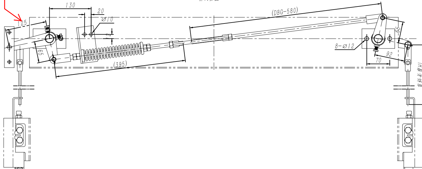
80010812 OX-210BTX 联动机构 (C=174,L3=200) DBG=1180(第二、三象限) 摇臂孔距105 中英文 海宁欧立 P1-2
