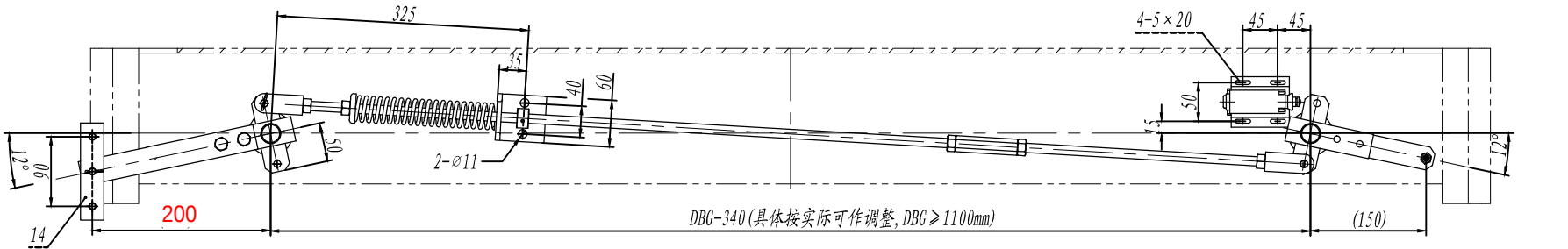
80010803 OX-188BT安全联动机构(提拉板孔距200)DBG=1440 C=220 L3=200 中英文 中都国脉 P1-2
