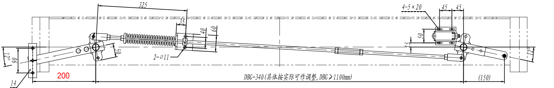
80010802 OX-188BT安全联动机构(提拉板孔距200)DBG=1740 C=220 L3=200 中英文 中都国脉 P1-2
