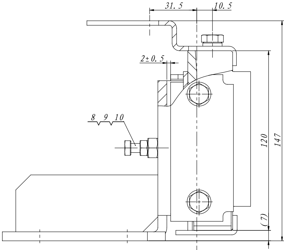
80010692 OX-029导靴(A03) 16mm RAL7037灰色 全英文 合肥蒂博
