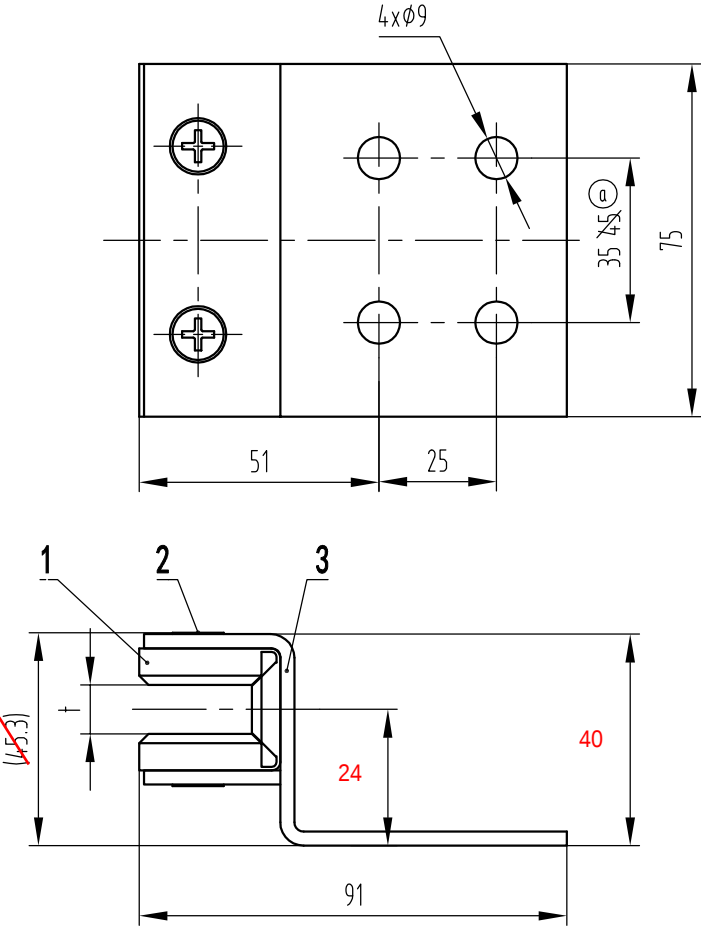
80010461 OX-310T导靴（特制）10mm 中英文 杭州西奥 P1-3
