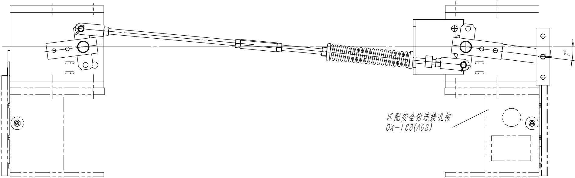
80010377 OX-188DT安全制动装置（左置）DBG=见备注 本色RAL6005 中英文 大连伊通
