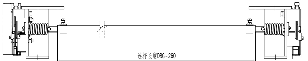
80010228 0X-210BZ安全钳联动机构(220) DBG=1780 蓝色RAL5015 中英文 韦伯电梯
