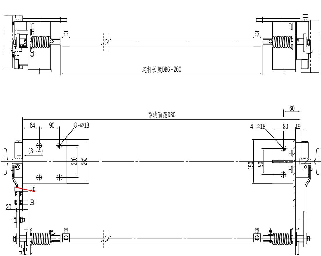
80010228 OX-210BZ安全钳联动机构(220) DBG=见备注 蓝色RAL5015 中英文 韦伯电梯
