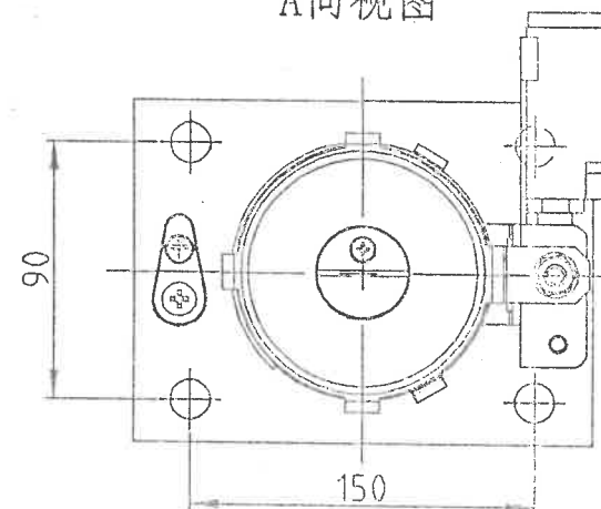
A向视图
