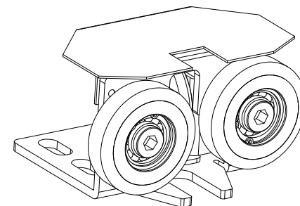
G01、G02三维模型
