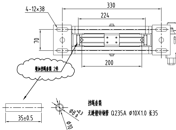
A向视图
