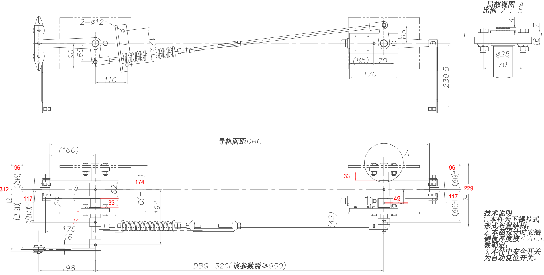
80009405 OX-188T安全联动机构 DBG=见备注 C=174 L3=210 中英文 华夏电梯 P1-4
