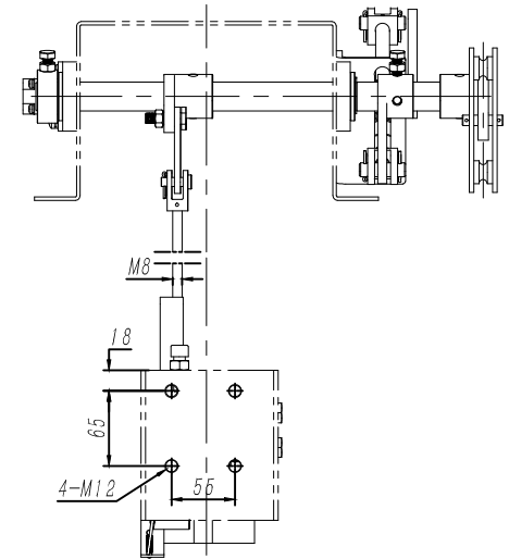
第1.4象限示意
