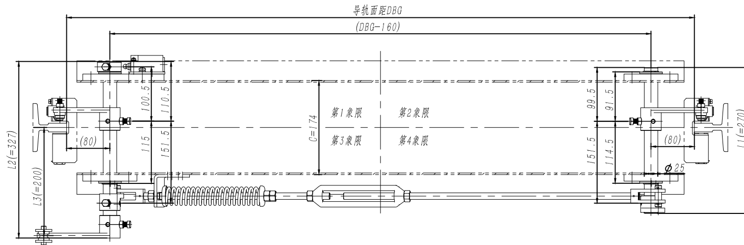
80009334 OX-210BTX联动机构 (C=174,L3=200)DBG=1180 (第二、三象限) 摇臂孔距105 中英文 海宁欧立 P1-2
