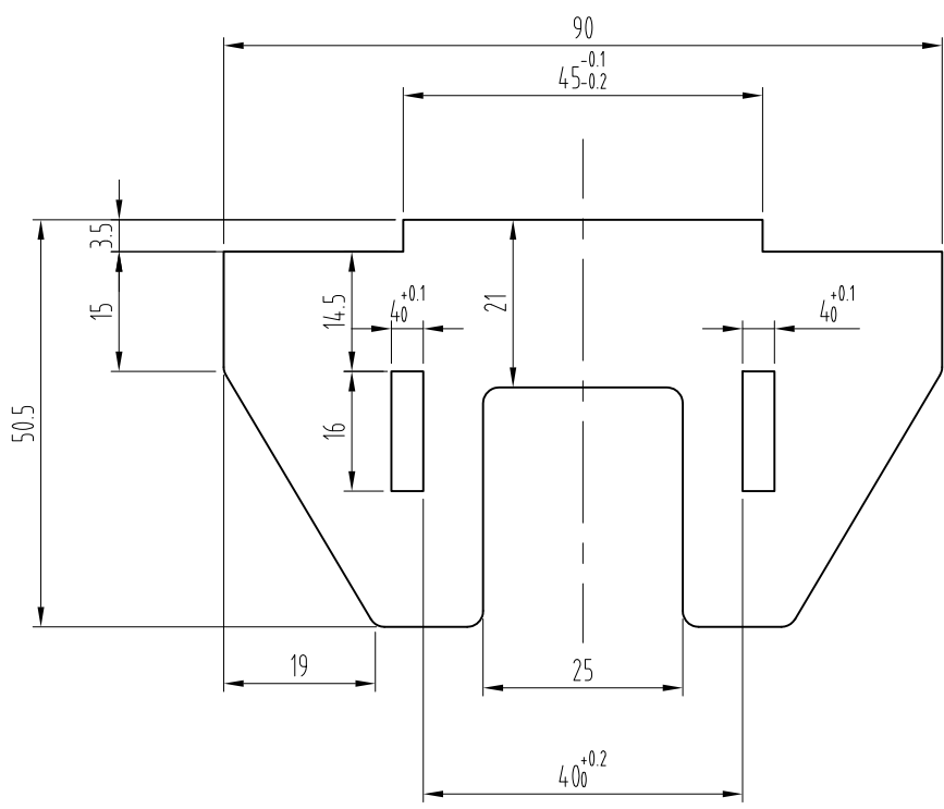
80009295 OX-310TX导靴 10mm 中英文 杭州西奥 P4
