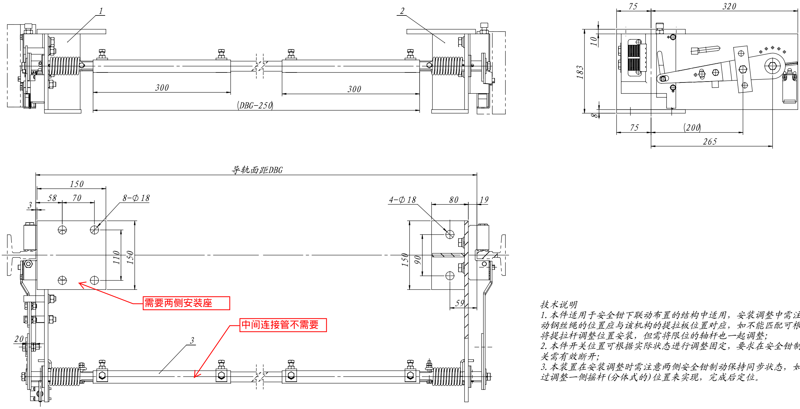
80009256 0X-210BZ安全钳联动机构(安装座) 本色RAL6005 中英文 德森克
