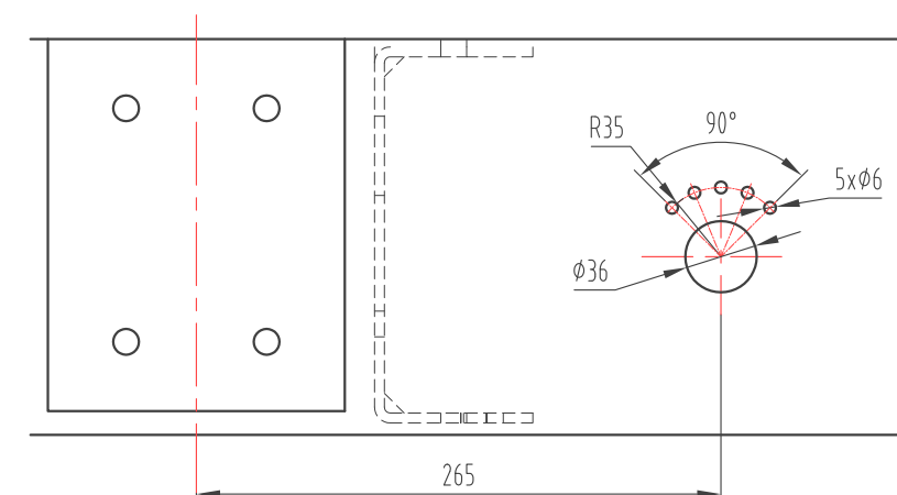
开孔示意图
