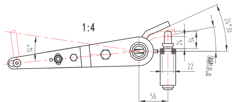
开关安装示意
