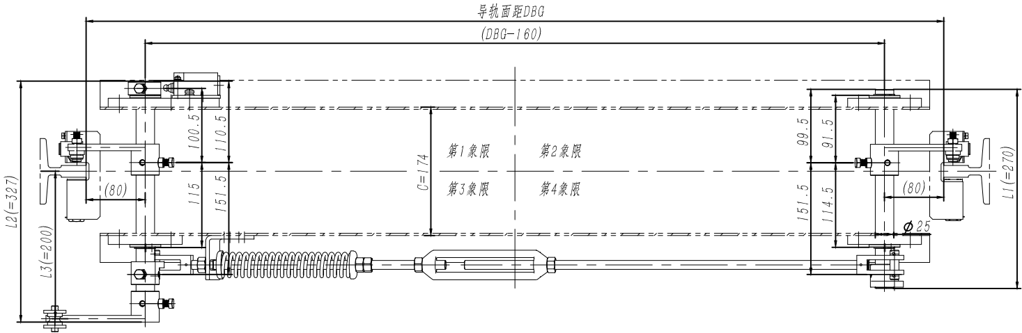
80009155 OX-210BTX联动机构 (C=174,L3=200)DBG=850 (第二、三象限) 摇臂孔距105 中英文 海宁欧立 P1-2
