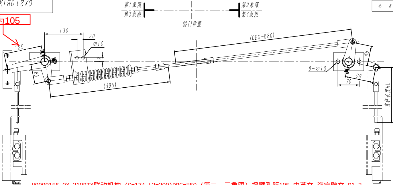
80009155 OX-210BTX联动机构 (C=174,L3=200)DBG=850 (第二、三象限) 摇臂孔距105 中英文 海宁欧立 P1-2
