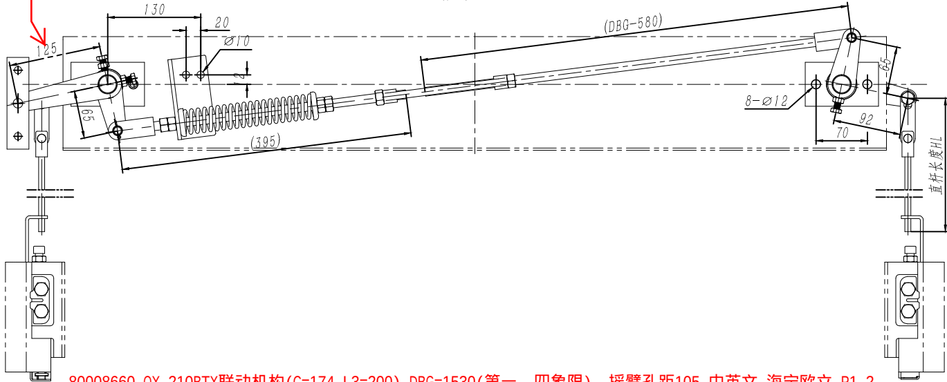
80008660 OX-210BTX联动机构(C=174,L3=200) DBG=1530(第一、四象限) 摇臂孔距105 中英文 海宁欧立 P1-2
