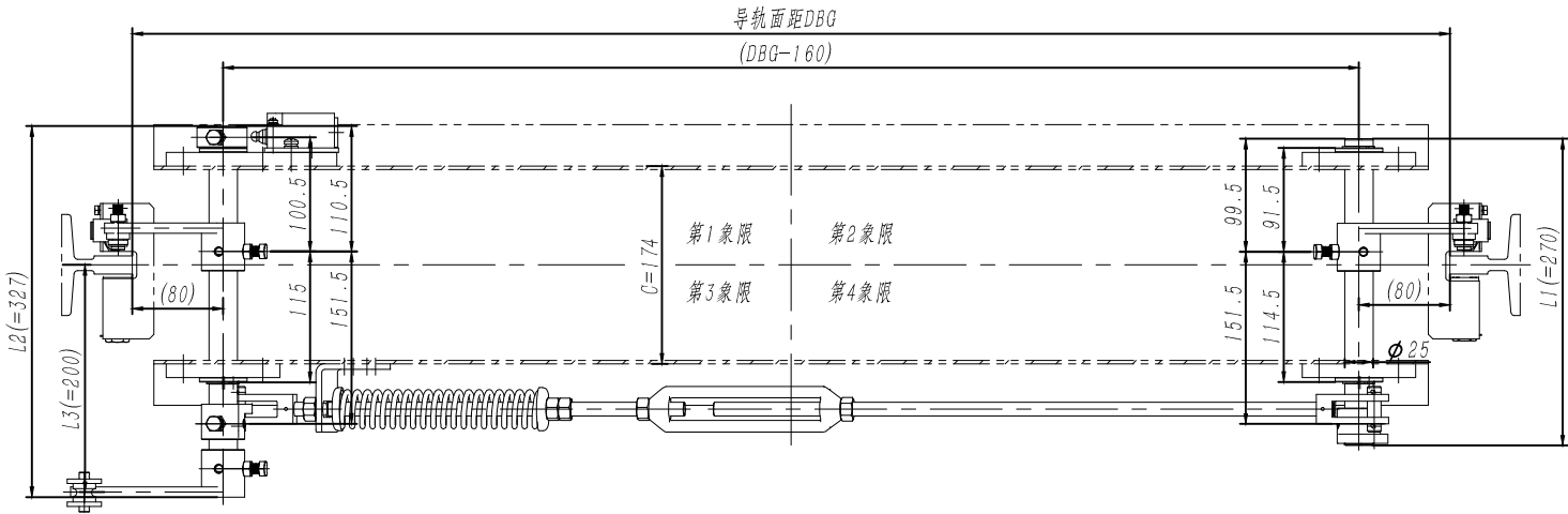
80008660 OX-210BTX联动机构(C=174,L3=200) DBG=1530(第一、四象限) 摇臂孔距105 中英文 海宁欧立 P1-2
