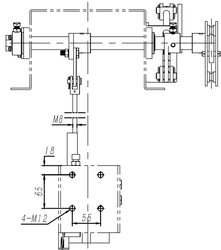
第1.4象限示意
