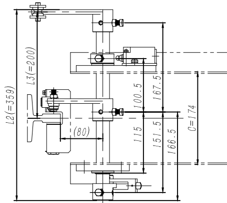
第1.4象限示意
