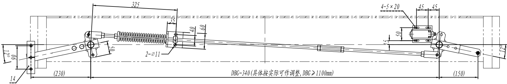
80007314 OX-188BT(C=158,A=200)安全联动机构 DBG=1710 中英文 帝奥电梯
