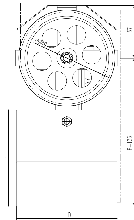
80007265 OX-300涨紧装置(240-90-200-44) 240-6 重晶石18kg 灰色RAL7037 中英文 怡达快速 P1-2
