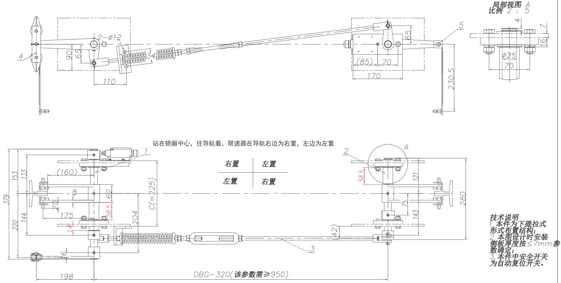
80006898 OX-188T安全联动机构(右置) DBG=1460 C=225 L3=220 中英文 江苏菱智 P1-5
