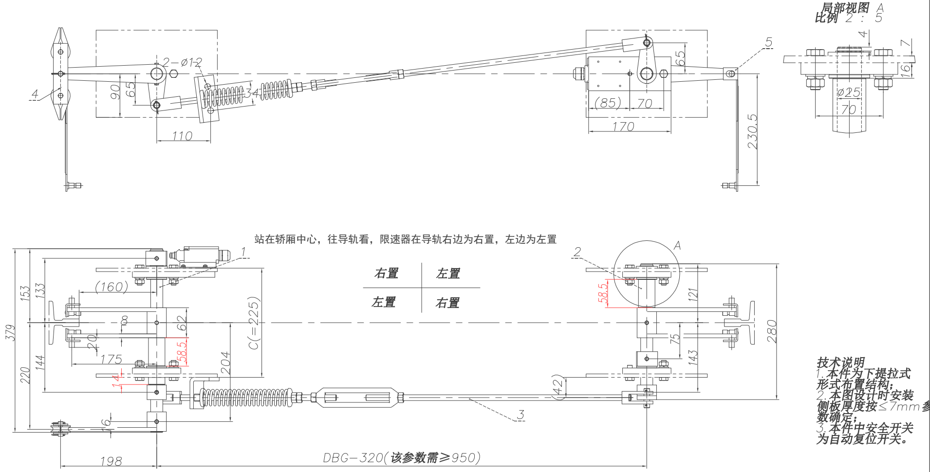
80006766 OX-188T安全联动机构(左置) DBG=1560 C=225 L3=220 中英文 江苏菱智 P1-5
