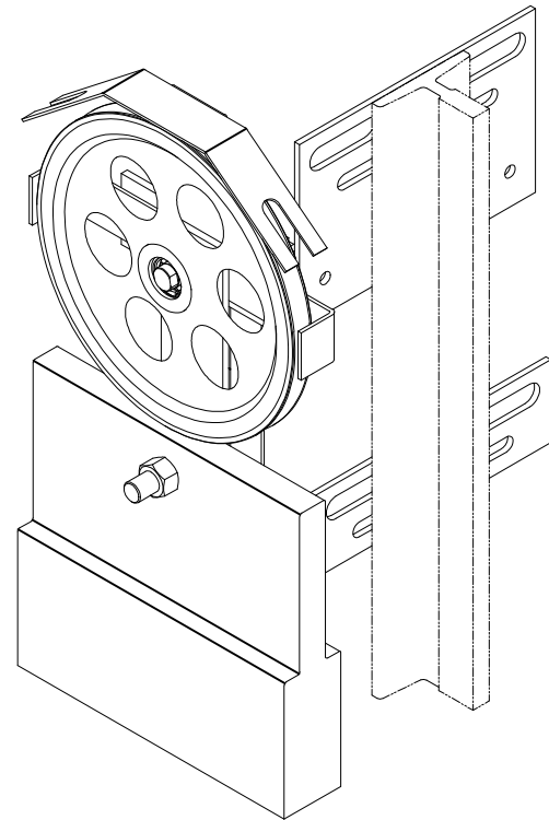
80003113 OX-300涨紧装置(240-90-240-50 T114) P1-2 240-8 铸铁18kg 本色RAL6005 中英文 东南电梯
