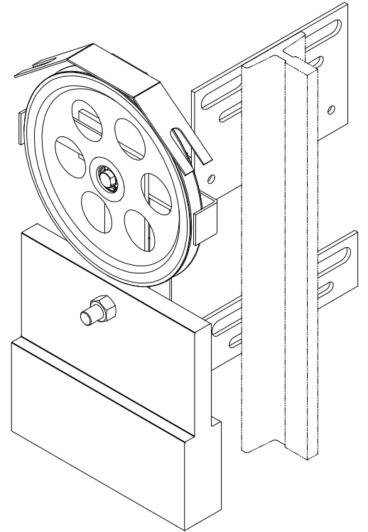
80003113 OX-300涨紧装置(240-90-240-50 T114) P1-2 240-8 铸铁18kg 本色RAL6005 中英文 东南电梯
