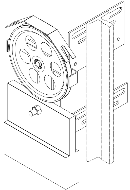
80002899 OX-300涨紧装置(240-90-240-50 T114) P1-2 240-8 重晶石18kg 本色RAL6005 中英文 东南电梯
