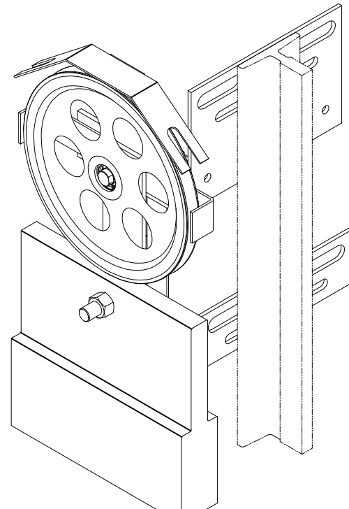
80002253 OX-300-TLW涨紧装置 240-8 P1-2 重晶石30kg A=220 B=82 本色RAL6005 中英文 苏州台菱
