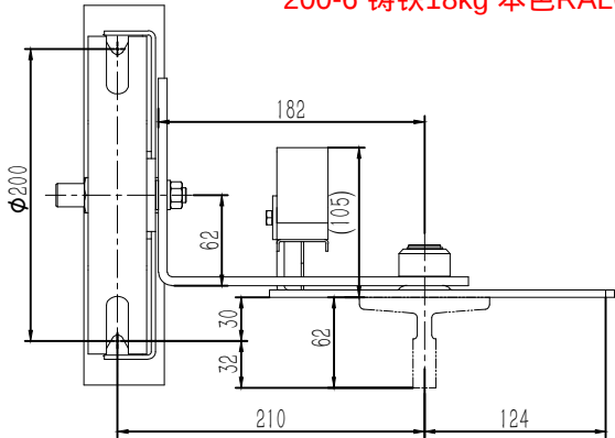
80002121 OX300涨紧装置(200-90-210-30) P1-2 200-6 铸铁18kg 本色RAL6005 中英文 苏州帝奥
