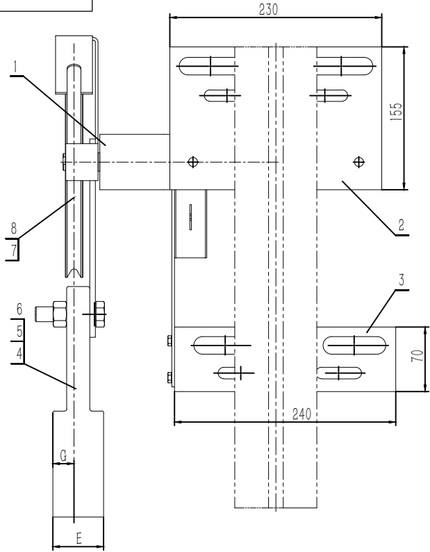
80002121 OX300涨紧装置(200-90-210-30) P1-2 200-6 铸铁18kg 本色RAL6005 中英文 苏州帝奥
