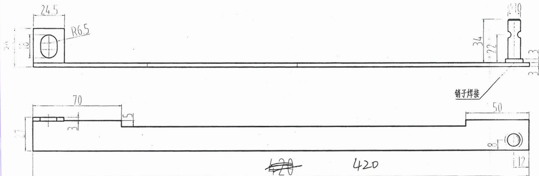
80002079 OX-188T.5提拉杆 L=420 (左右各二) 恒达富士
