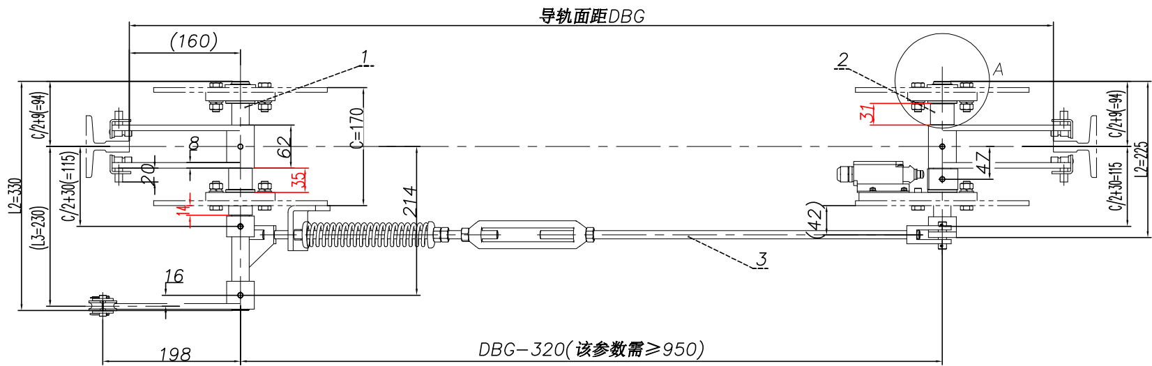
80002070 OX-188T安全联动机构 P1-6 DBG=1350 C=170 L3=230 中英文 福德斯
