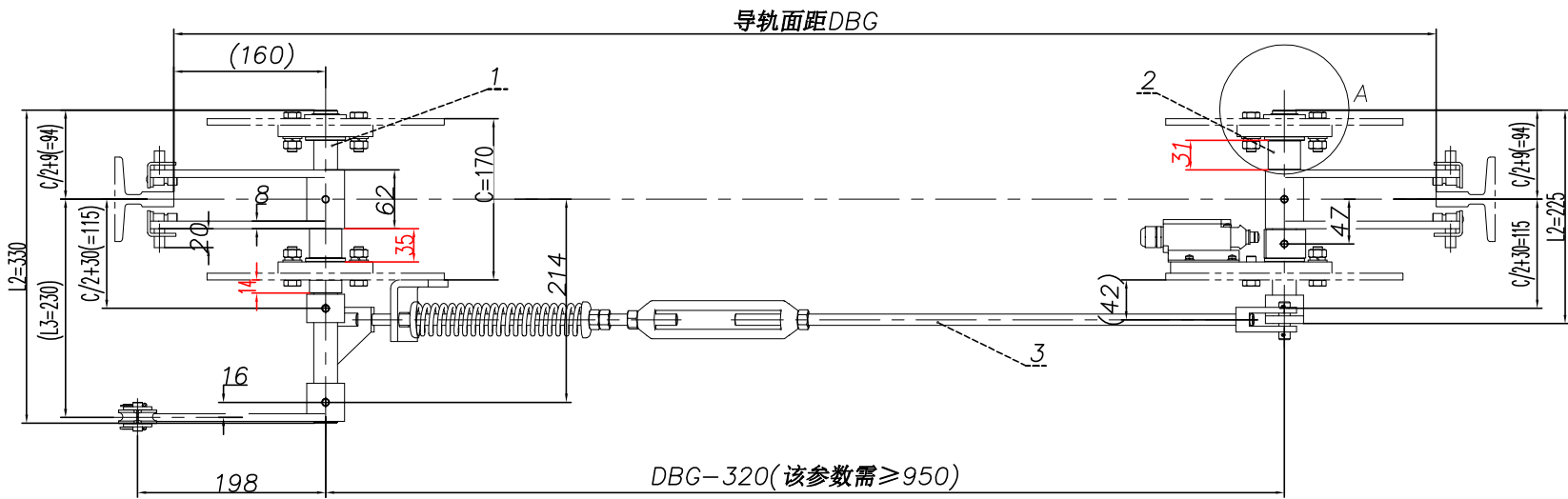
80002043 OX-188T安全联动机构 P1-6 DBG=1300 C=170 L3=230 中英文 福德斯
