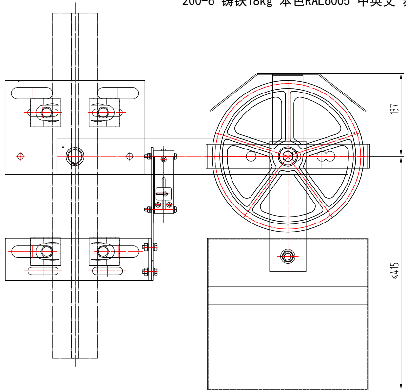
80001710 0X-300涨紧装置 (200-135-220-40) P1-2 200-6 铸铁18kg 本色RAL6005 中英文 苏州菱奥
