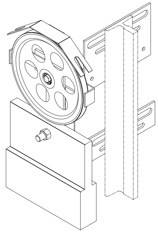
80001374 OX-300涨紧装置(V5) 广东奥菱 P1-2 200-6 铸铁30kg 本色RAL6005 中英文
