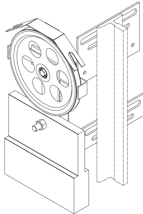
80001339 OX-300涨紧装置 东南电梯 P1-2 240-8 本色RAL6005 铸铁18kg 中英文
