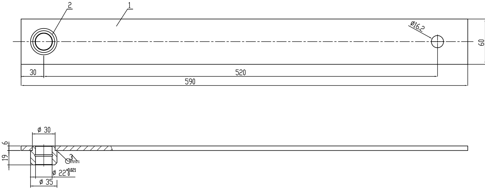
80001210 摇杆组件 (A=520) 本色RAL6005 通用电梯 P2-2
