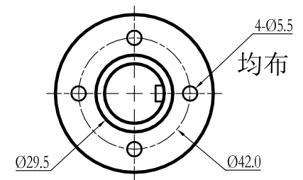
剖面B-B
