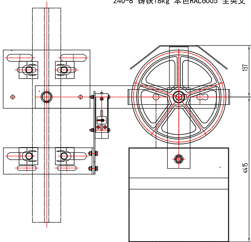
80001129 0X-300涨紧装置 (240-135-200-25) 林肯电梯 P1-2 240-8 铸铁18kg 本色RAL6005 全英文
