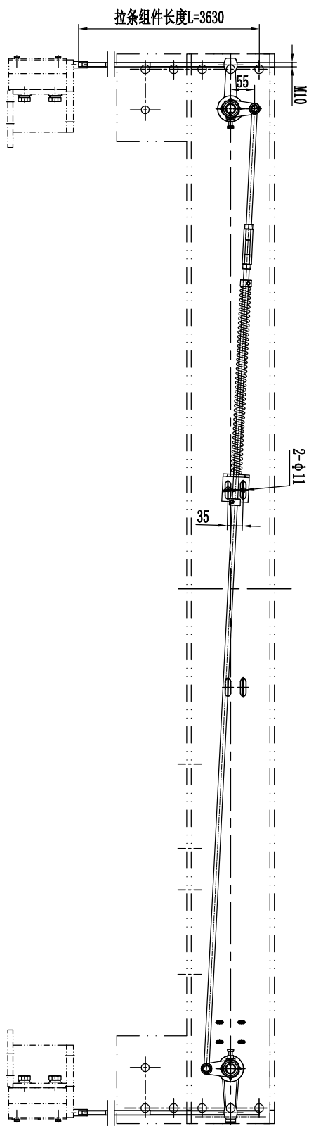
80000945 OK-288T 安全联动装置 沈阳远大 P2-2 DB=2350mm C=230 L1=310mm L2=405mm L3=220mm HL(M10)=3630mm 4根(配UKS开关组件，不要钢丝绳连接件)
