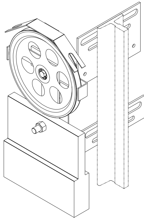
80000771 OX-300(240-90-200-39) 涨紧装置 240-8 18kg(重晶石) 灰色RAL7037 中英文 苏州莱奥 P2-1
