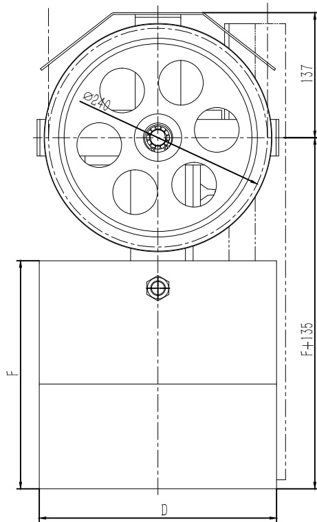
80000771 OX-300(240-90-200-39) 涨紧装置 240-8 18kg(重晶石) 灰色RAL7037 中英文 苏州莱奥 P2-1
