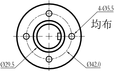
剖面B-B
