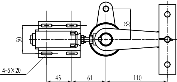
剖面A-A
