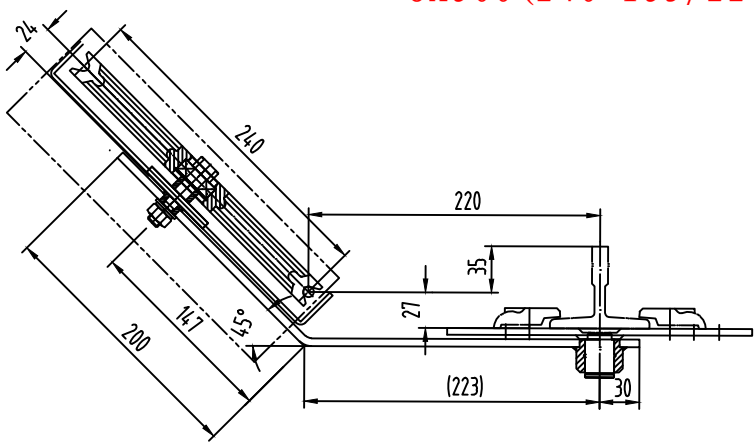
OX300(240-135/220-27) 涨紧装置 (本件可左右对称使用)
