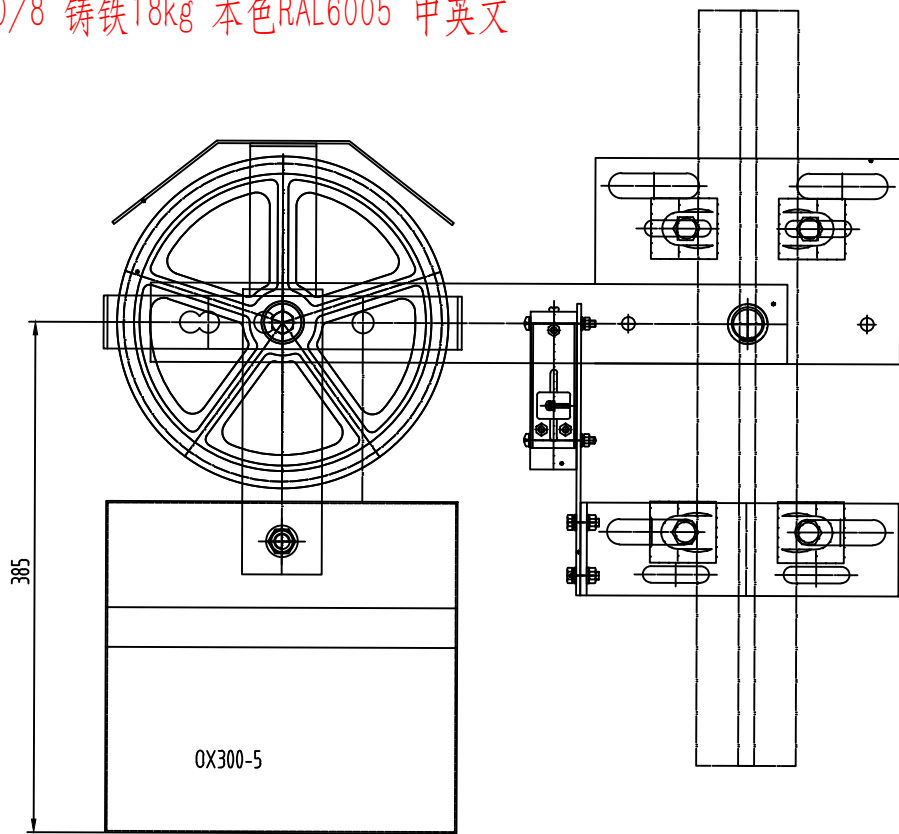
OX300(240-135/220-27) 涨紧装置 (本件可左右对称使用)
