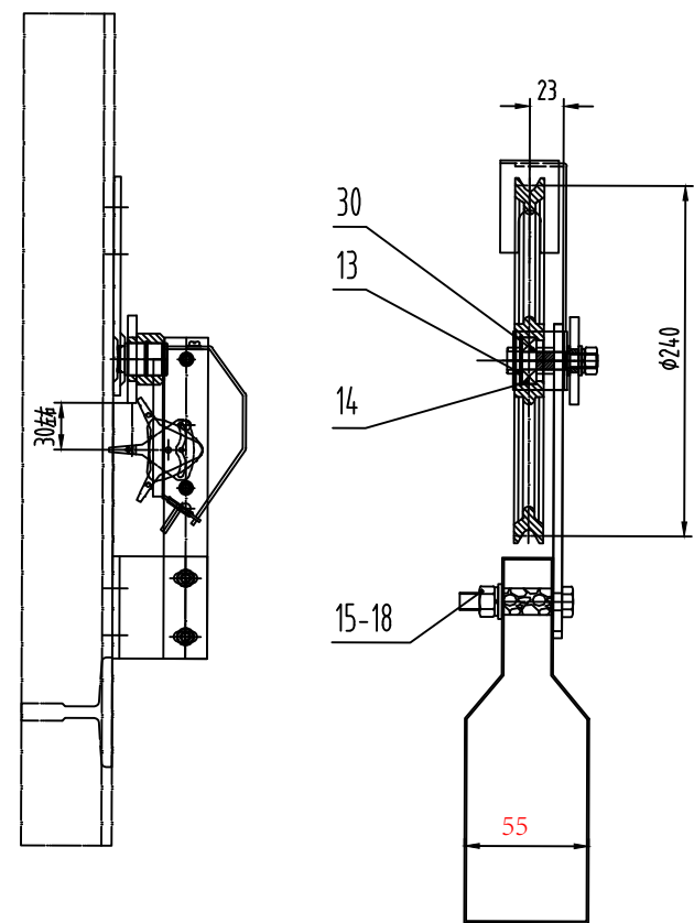
OX300(240-135/220-27) 涨紧装置 (本件可左右对称使用)
