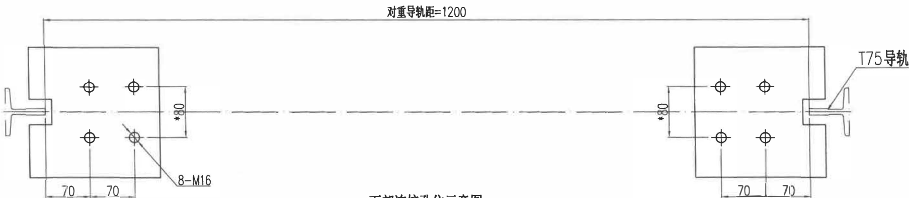
下部连接孔位示意图
